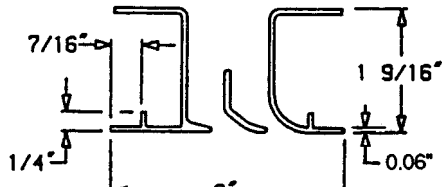
AG TYPE DIFFUSER (1-WAY)
